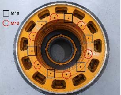
쉬브 635MM 하이브리드 635X30(M12 19MM)
