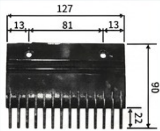
동양 LXW 블랙 YS013B578
