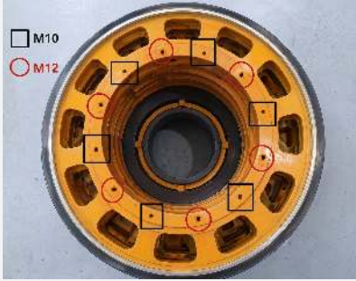
쉬브 587MM 하이브리드 587x330x30(M10,17MM) 587x330x30(M10,17MM)
