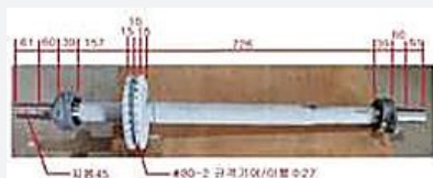
잭샤프트 (현대 호환제품)1200형
