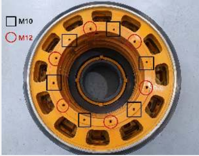
쉬브 587MM 하이브리드(우레탄) TPU 587x330x30(M10,17MM) 587x330x30(M10,17MM)
