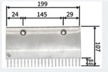
미쓰비시(중간) J651004b203 알 루미늄
