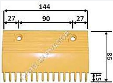
티센 무빙워크 SY3000000007488
