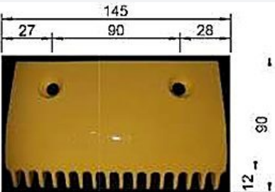
오티스 2L8316 일련번호 2L8316
