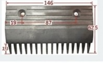
동양,티센스텝 LXW /실폭800 30/35도 알루미늄S655B609H02
