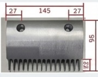
오티스 (줄무늬)
