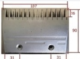
미쓰비시(중간) 751001B2020 알루미늄
