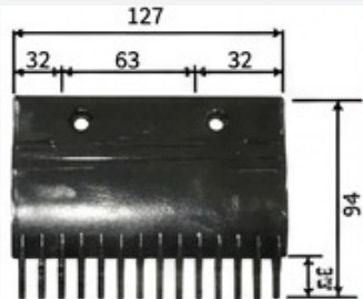
미쓰비시 HS017B313
