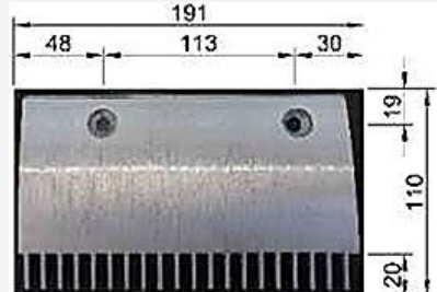
티센 9011 (티센벨리노)
