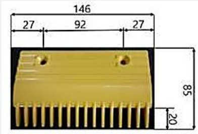
현대 HE655B013
