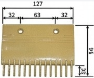
미쓰비시 YS017B313
