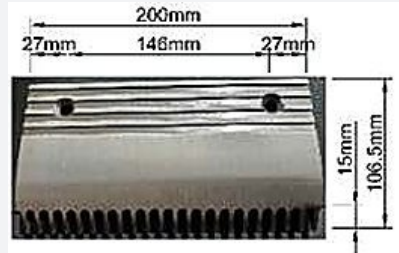
현대 C65500390H02 좌측 C65500390H03 우측
