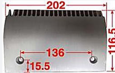
현대 655 B013H06
